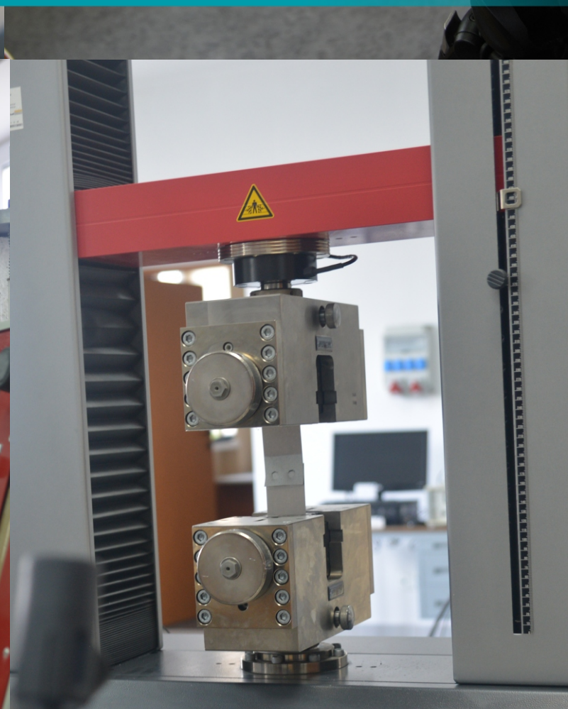
Uniwersalna maszyna wytrzymałościowa – laboratorium konstrukcji metalowych
