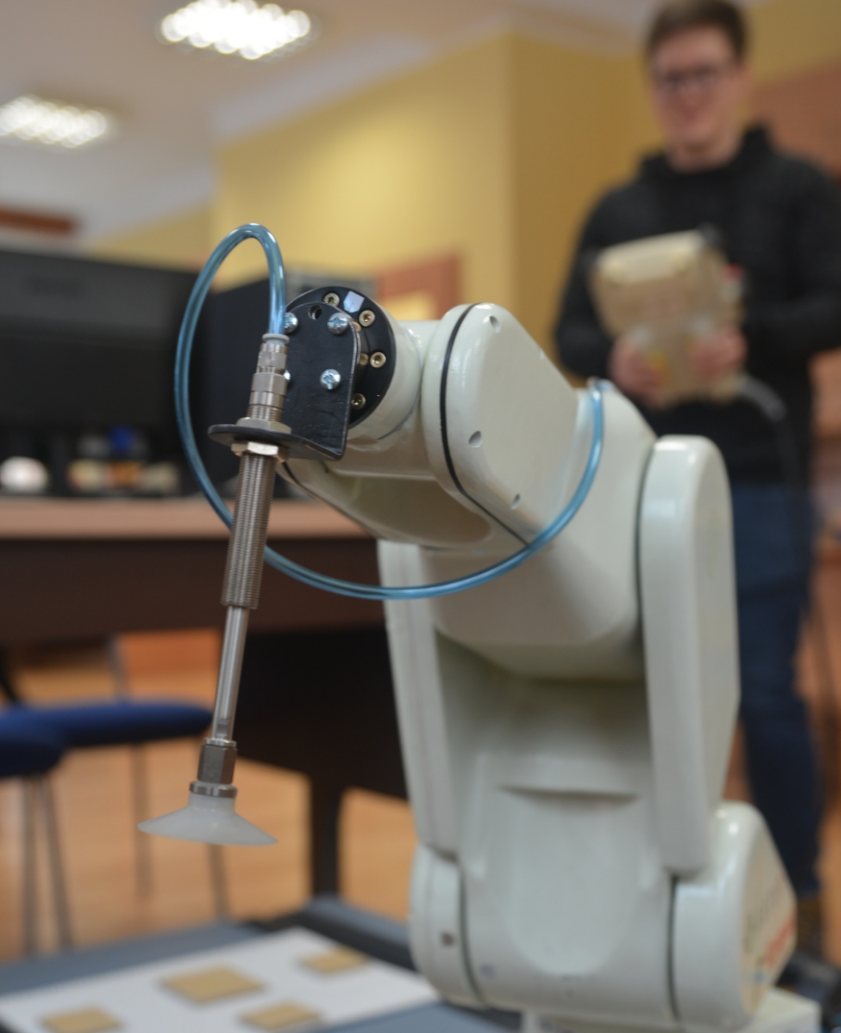
Manipulator elektromechaniczny z chwytakiem pneumatycznym robota przemysłowego Kawasaki – laboratorium robotyki
